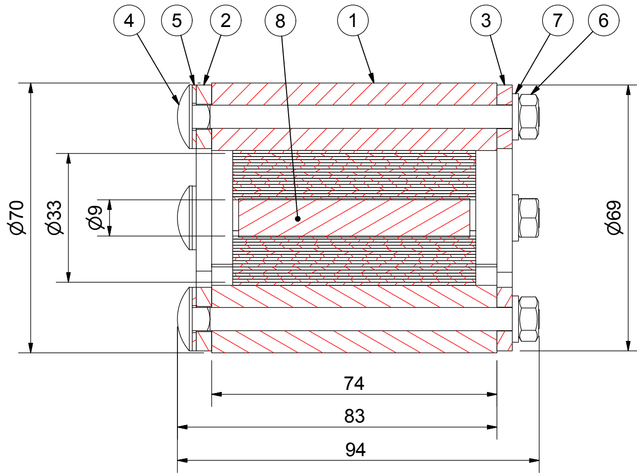
A-A ( 1 : 1 )
